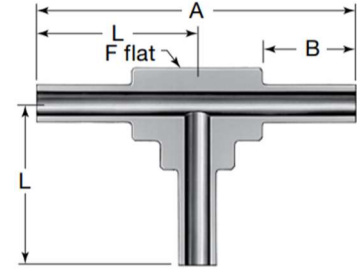
Tee
