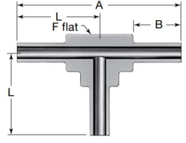
Tee
