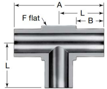
Tee
